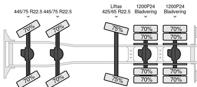
Mercedes-Benz 5044 Actros AK - 10x8 - Euro5 - Telligent 3 p...
